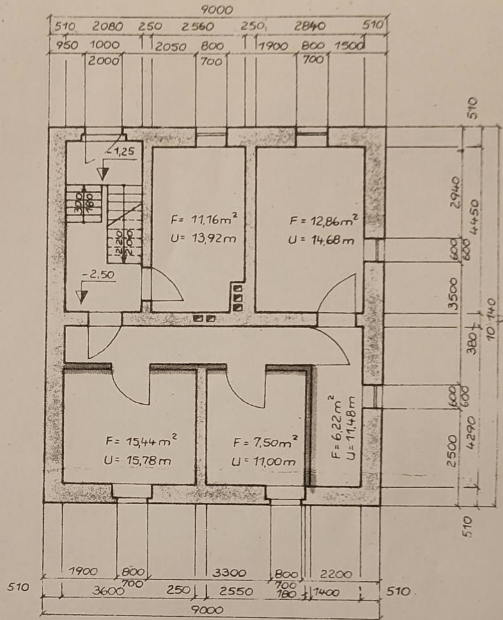
Kellergeschoß
