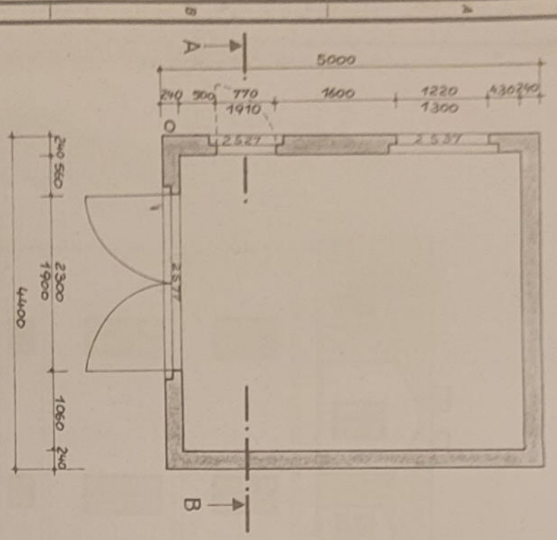
M 1:50
