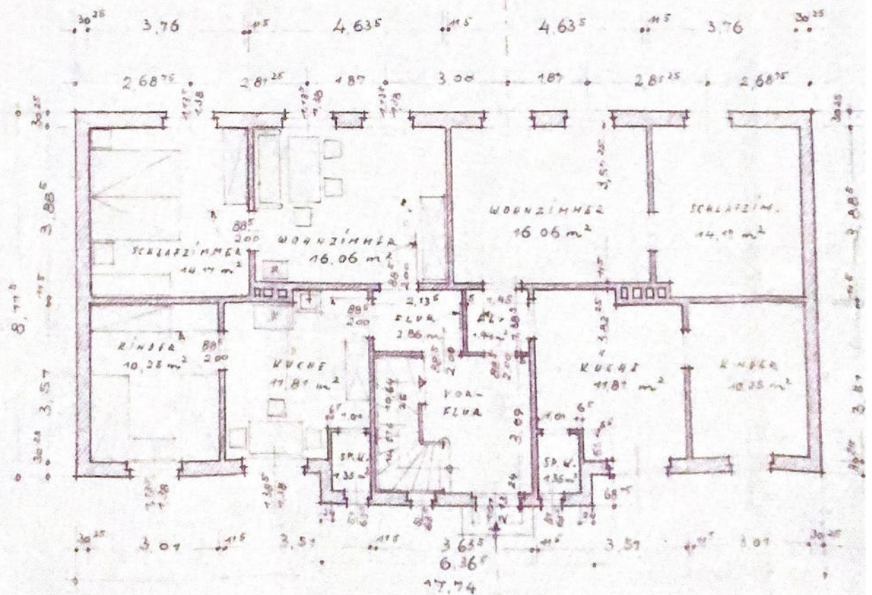
ERDGESCHOSS
