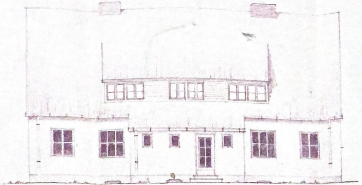
NORD-ANSICHT
