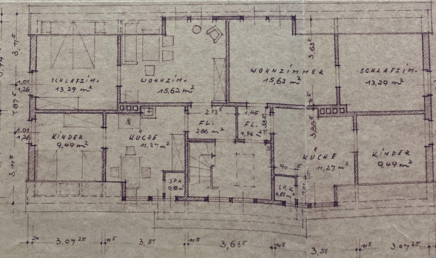
DACHGESCHOSS
