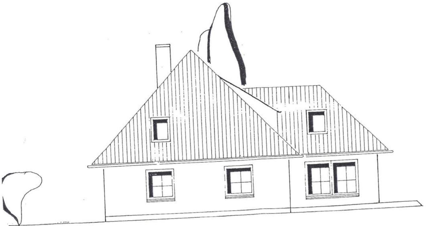
Westansicht
